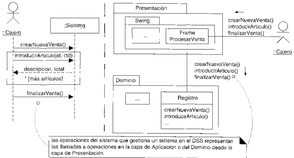
Figura 30.10. Operaciones del sistema en los DSSs y en función de las capas.
