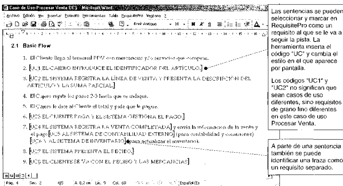
Figura 36.4. Etiquetado básico de frases de los casos de uso como requisitos.
