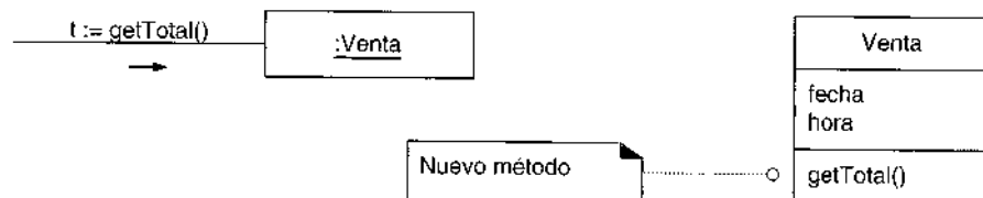
Figura 16.4. Diagramas de interacción y de clases parciales.
