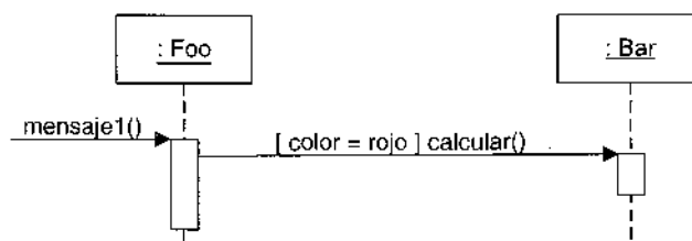
Figura 15.22. Un mensaje condicional.
