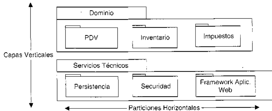
Figura 30.13. Capas y particiones.
