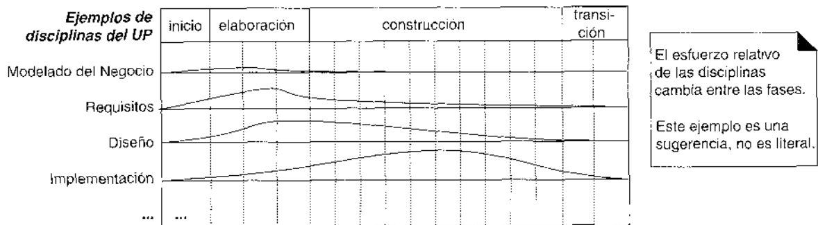
Figura 2.5. Disciplinas y fases.
