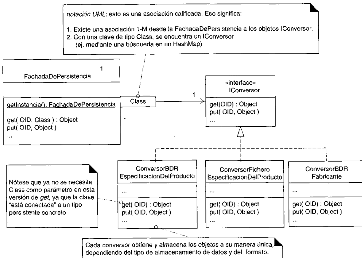
Figura 34.5. Conversores de bases de datos.
