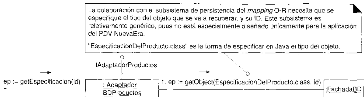
Figura 33.6. Colaboración con el subsistema de persistencia.
