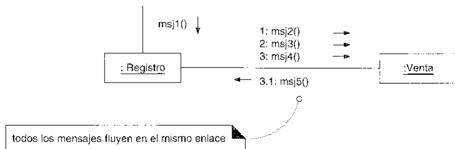
Figura 15.7. Mensajes.
