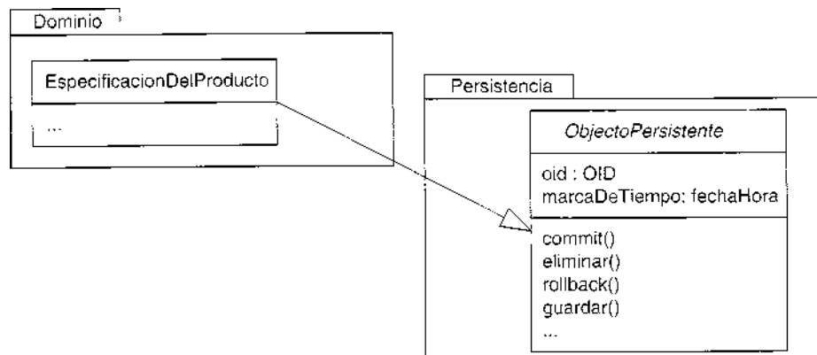
Figura 34.13. Objetos persistentes.
