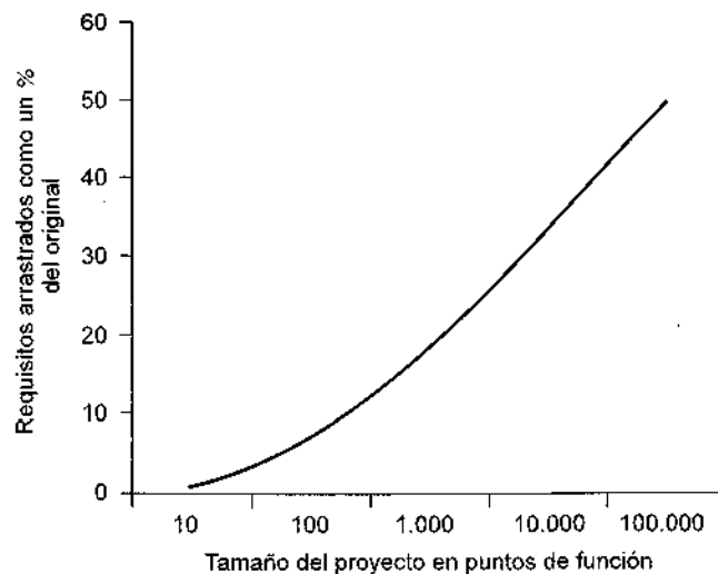
Figura 37.3. Los requisitos que cambian son una fuerza inevitable del desarrollo 2 .
