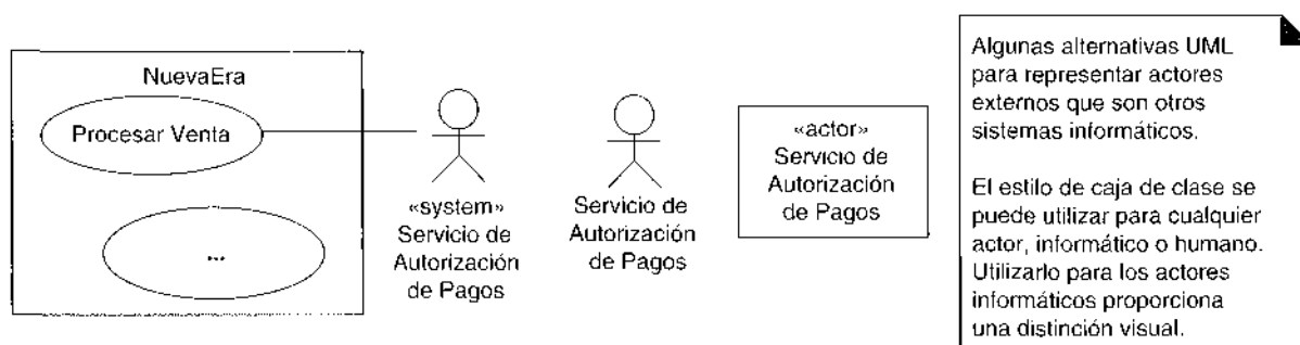
Figura 6.4. Notación alternativa para los actores.
