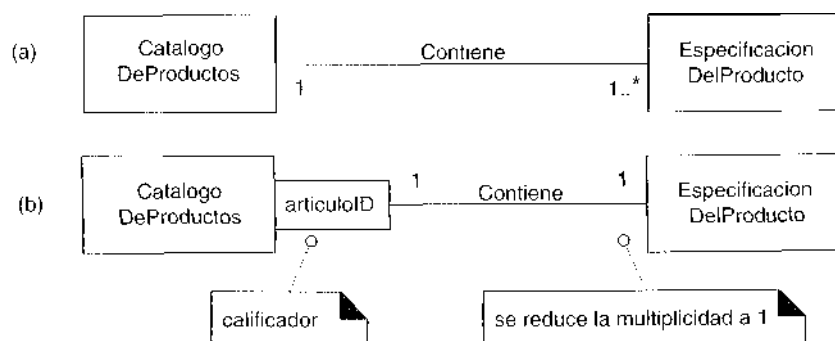
Figura 27.14. Asociación calificada.
