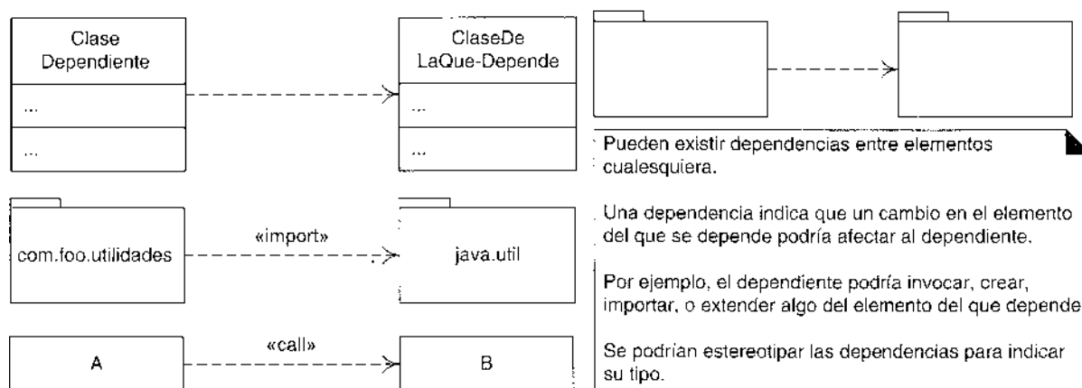
Figura 38.3. Dependencias.
