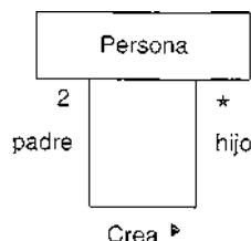
Figura 27.15. Asociación reflexiva.
