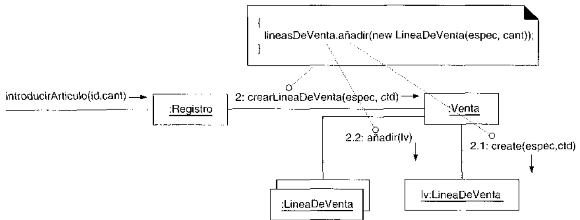
Figura 20.10. Método Venta—crearLineaDeVenta.
