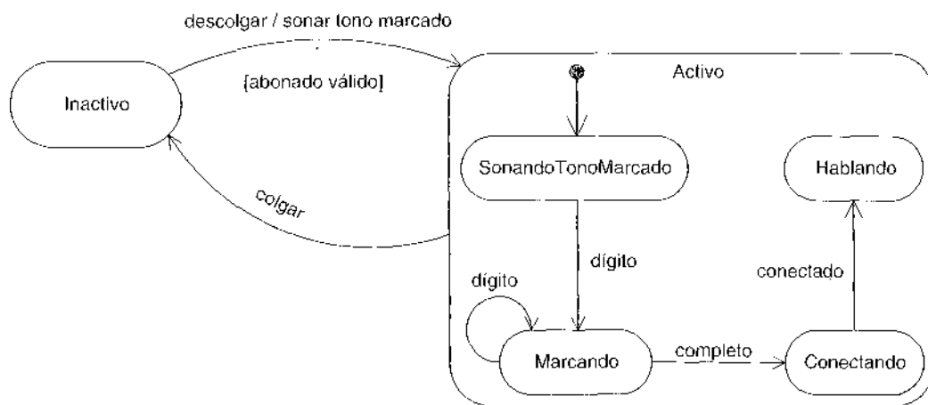
Figura 29.5. Estados anidados.
