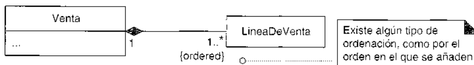
Figura 27.16. Elementos ordenados.
