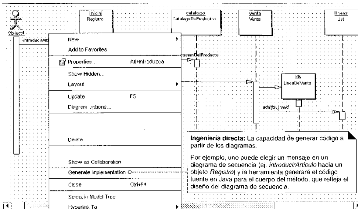
Figura 35.1. Ingeniería directa.
