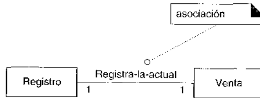
Figura 11.1. Asociaciones.
