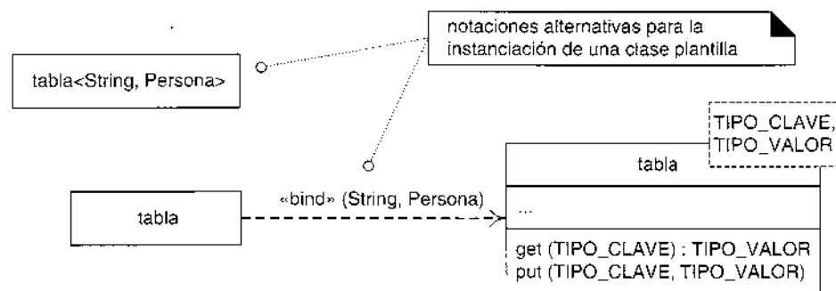
Figura 38.6. Clases plantilla.
