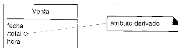
Figura 27.12. Atributo derivado.
