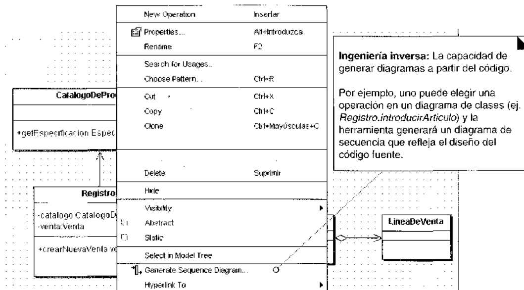
Figura 35.2. Ingeniería inversa.
