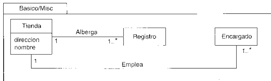
Figura 27.22. Paquete básico.
